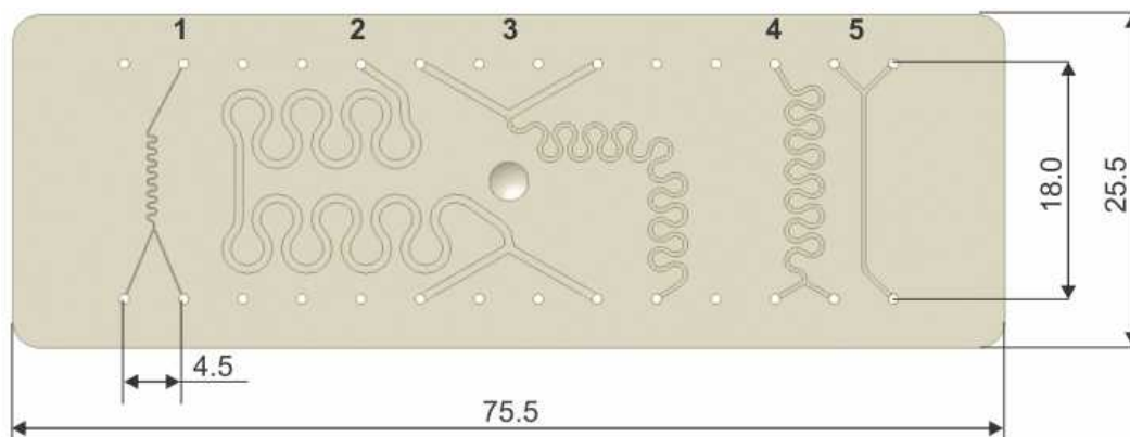
底面図 単位(mm)
